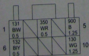
接天窗电机
